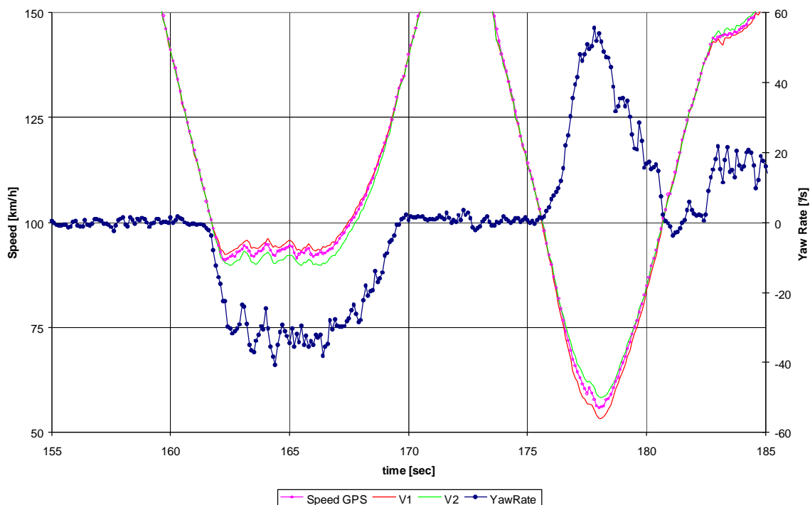
Figura 5. Particolare dell'acquisizione: i segnali di velocità in due curve opposte.
