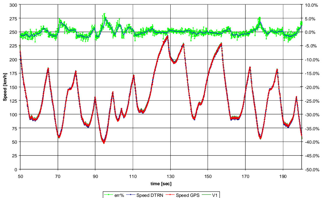
Figura 4. sovrapposizione dei profili di velocità acquisiti con il sensore ottico (speed DTRN), con la ruota fonica (V1) e calcolati sulla base della misura GPS.
