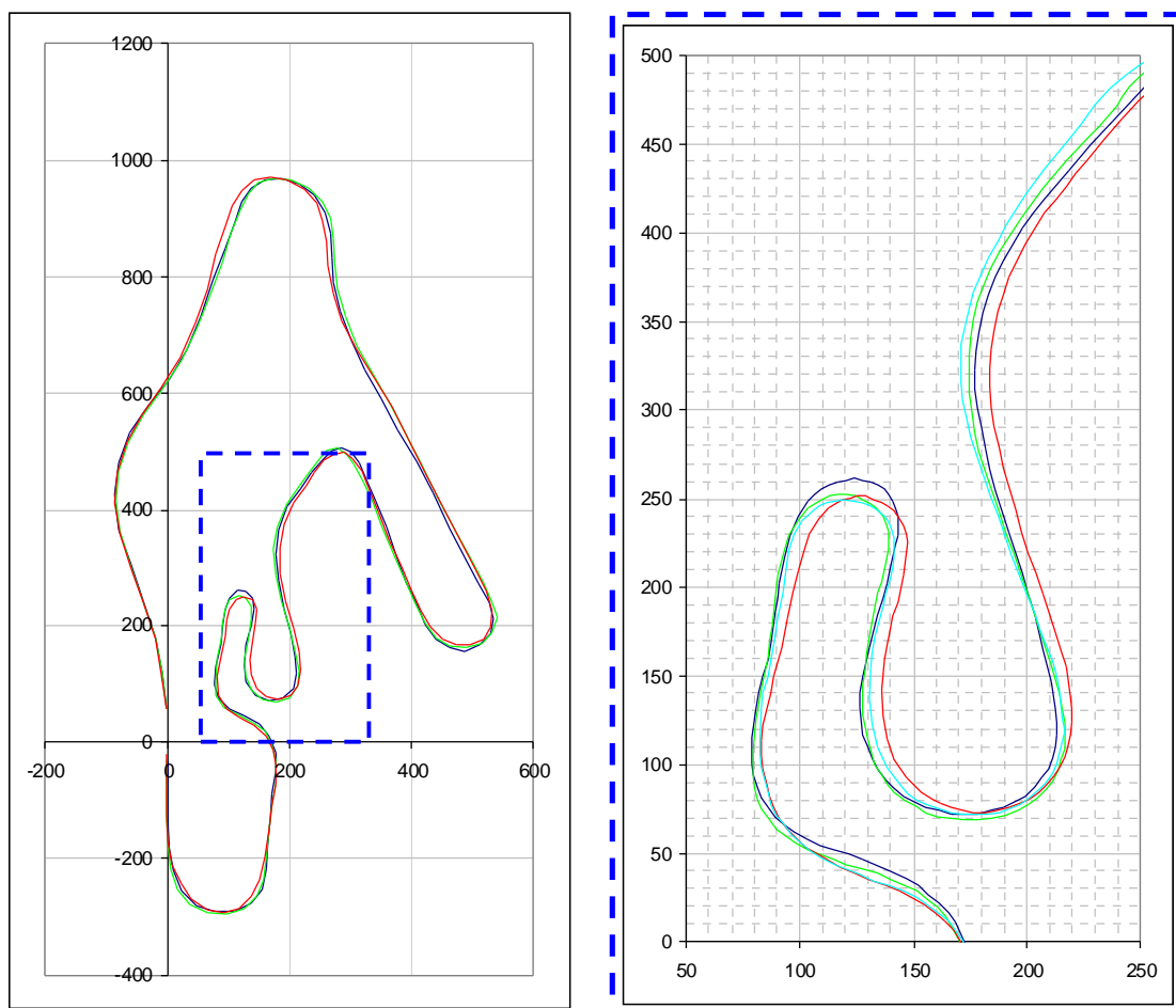
Figura 2. ricostruzione del tracciato attraverso i sensori ruota fonica e l'accelerometro (particolare a destra).
