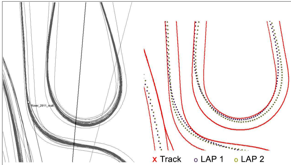
Figura 3. Dettaglio della curva “Semaforo”: rilevamento dei bordi pista e traiettorie nella sessione di prove (sinistra), estrazione di due giri consecutivi (destra).
